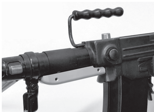
Figura 21: Paramano del F ass 57
