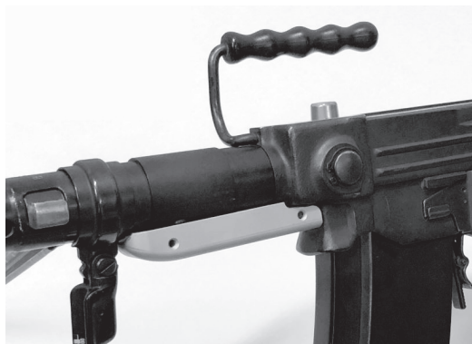
Figure 21: Garde-main pour F ass 57
