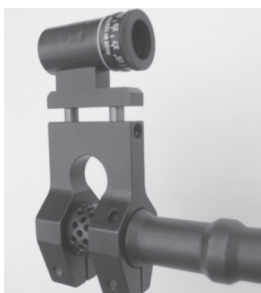
Figura 15: Portamirino come prolungamento della linea di mira (montaggio sul freno di bocca), diversi modelli
