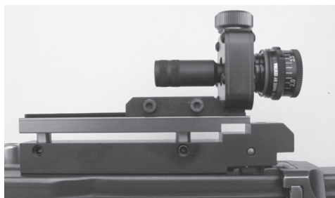
Figura 16: Supporto dell'alzo per il F ass 57 per il montaggio di comuni alzi circolari resistente agli urti e/o contraccolpi – rinculo, diversi modelli
